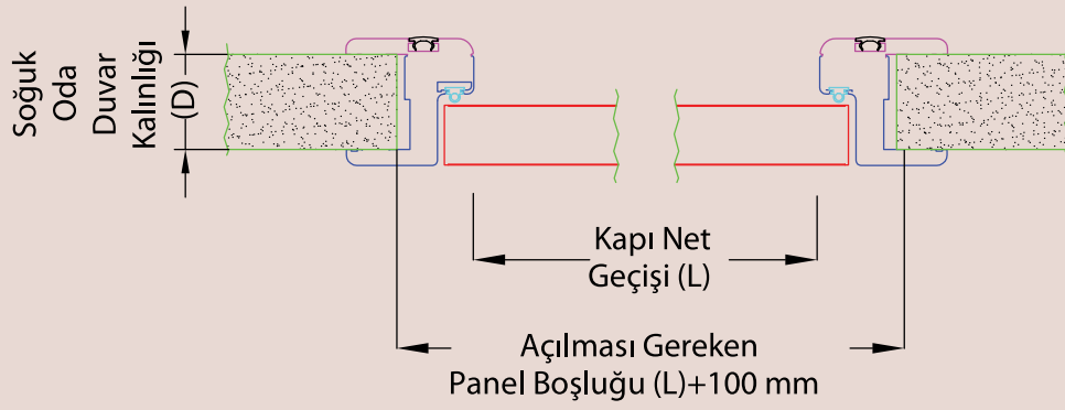
TCP KASA (TEK KANAT) DİK KESİT
